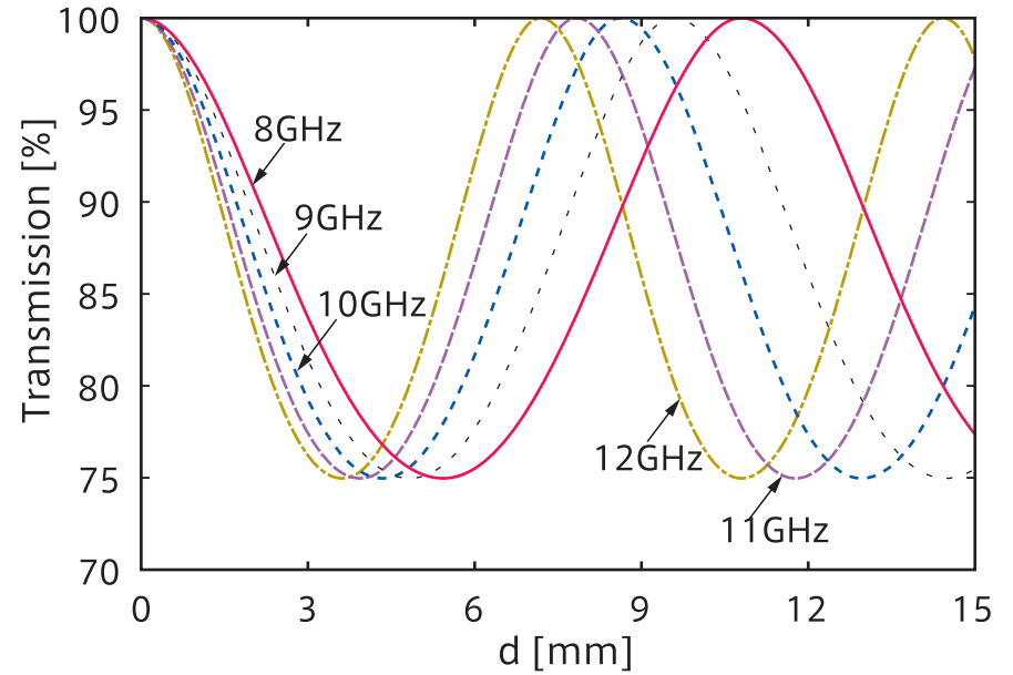
誘電率 \epsilon_r = 3.0 (1.25倍発泡)
