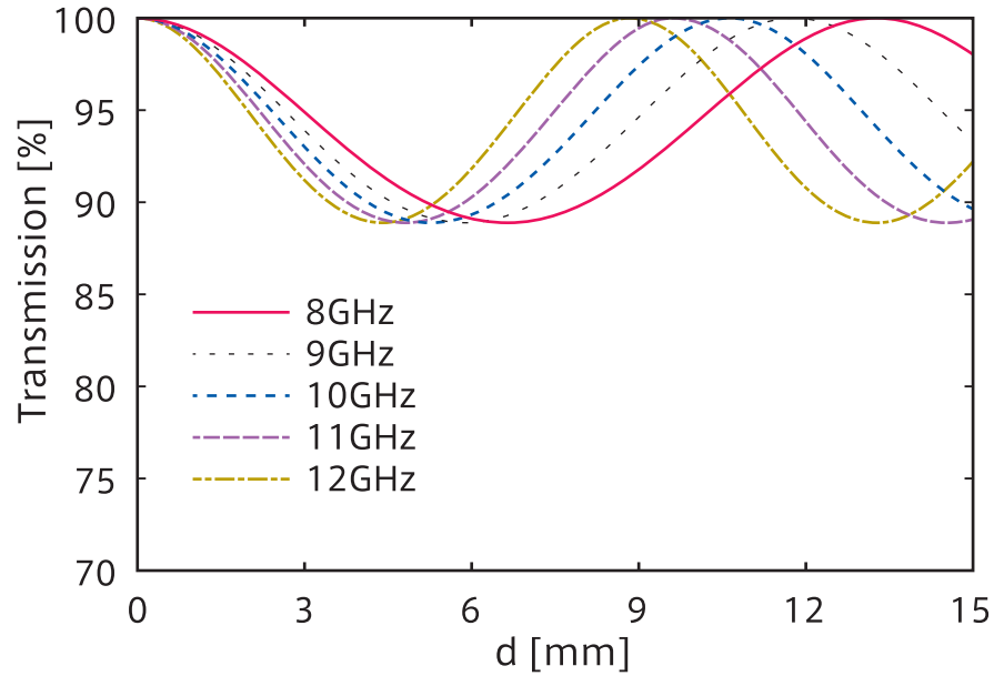
誘電率 \epsilon_r = 2.0 (2倍発泡)
